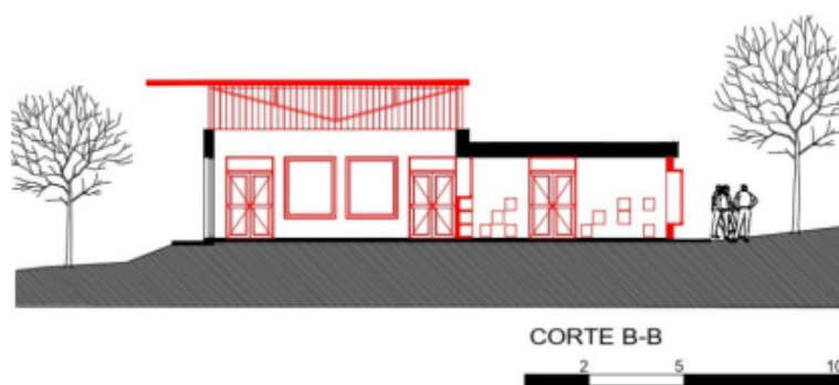
Imagen 2: Aula abierta corte B-B
