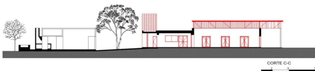
Imagen 3: Aula abierta corte C-C.
